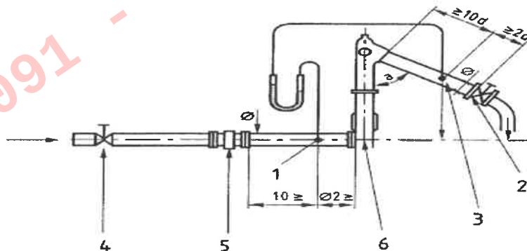
Şekil 4. Akış Karakteristiği Test Düzeneği Örneği (TS EN 14384 Şekil-3)
